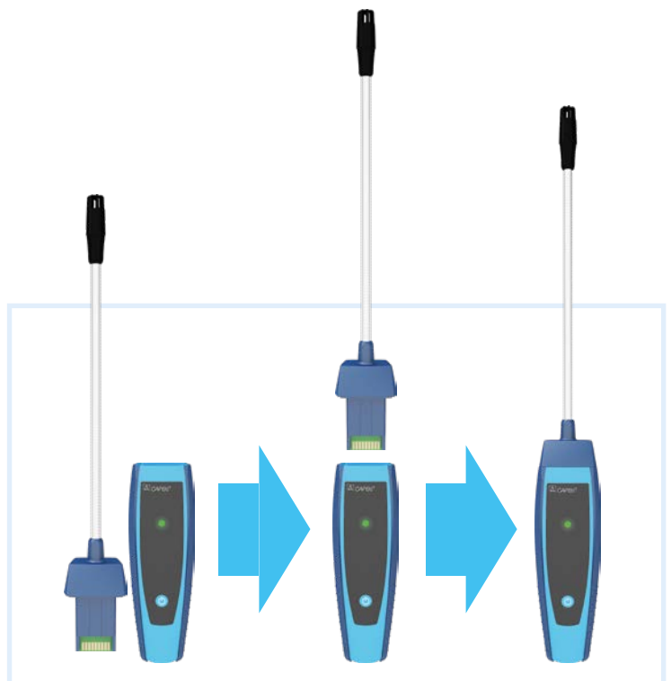
Modulares Wechselsystem
